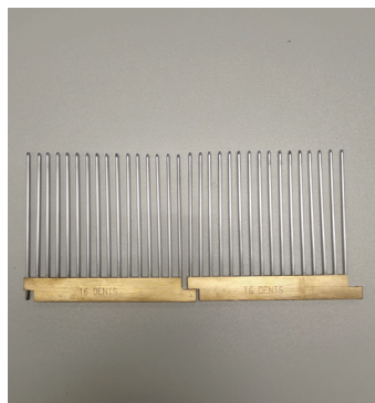
Peines urdidor (100 ml). Warper combs (100 ml).
