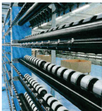
Guía hilos elastómero GRE. Threads guide for elastomeric yarn GRE.
