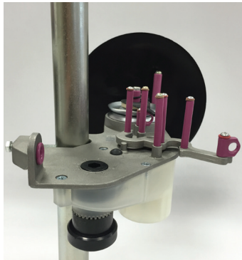
Tensor hidráulico desde 80 hasta 3000 dtex Hydraulic tensioner from 80 to 3000 dtex
